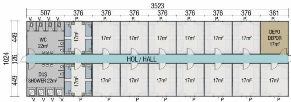
Zemin Kat Planı (360 m 2 )
