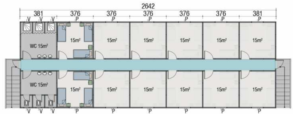
1. Kat Planı (237 m 2 ) First Floor
