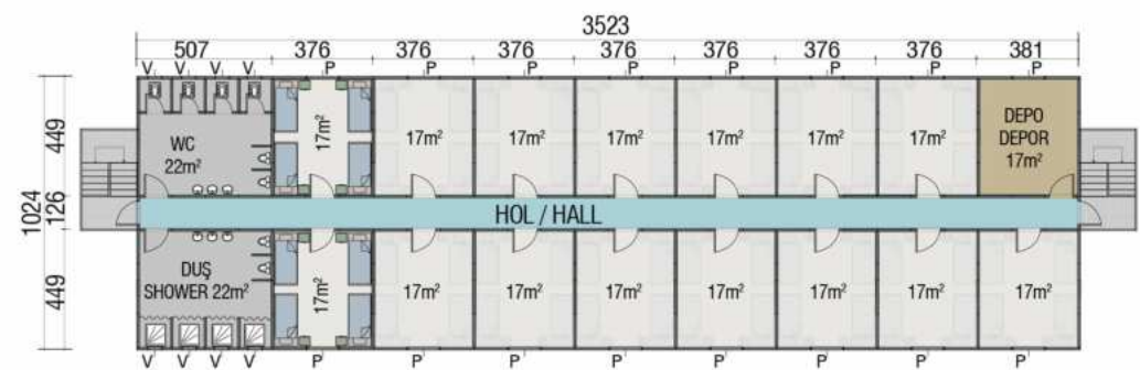
1. ve 2. Kat Planı (360 m 2 )
