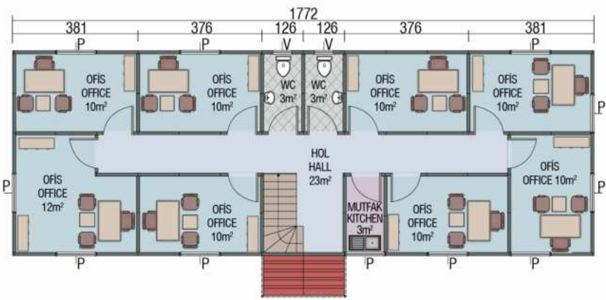
1. Kat Planı (159 m 2 ) First Floor
