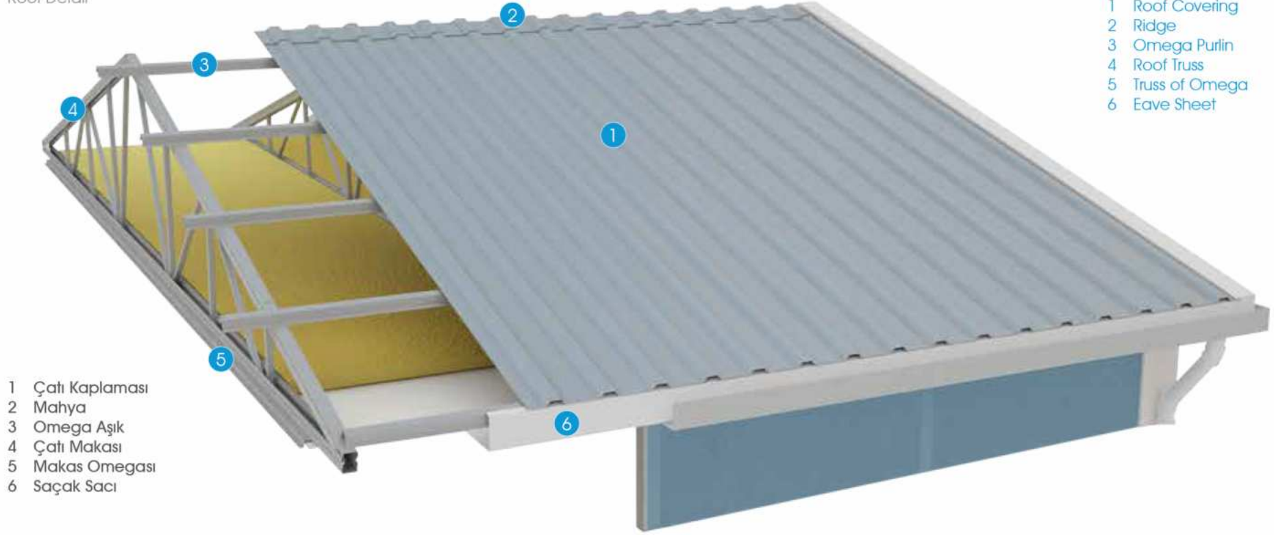
Çatı Detayı Roof Detail
