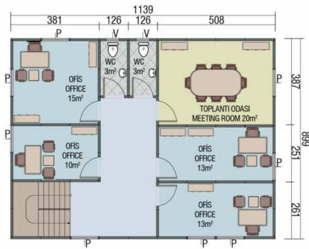
1. Kat Planı (102 m 2 ) First Floor
