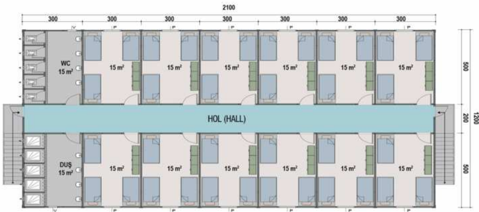
Üst Kat Planı / First Floor (252m 2 )
