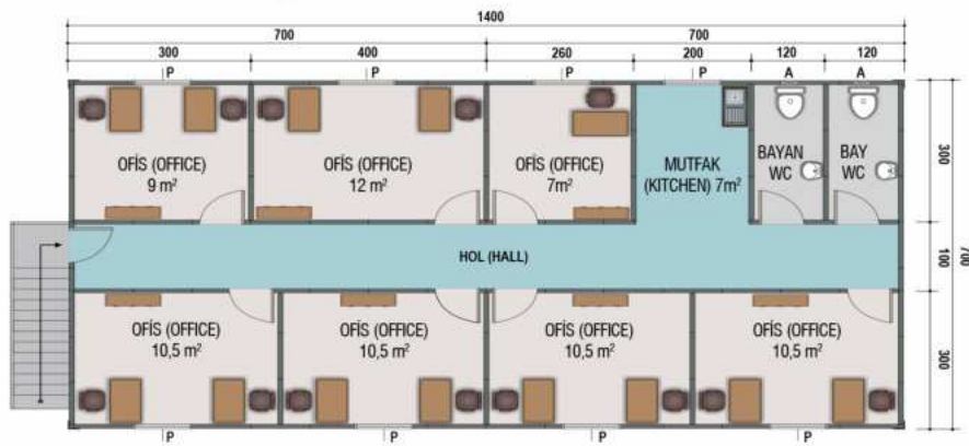
Üst Kat Planı / First Floor (98m 2 )
