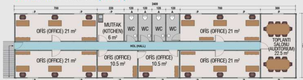
Üst Kat Planı / First Floor (180m 2 )
