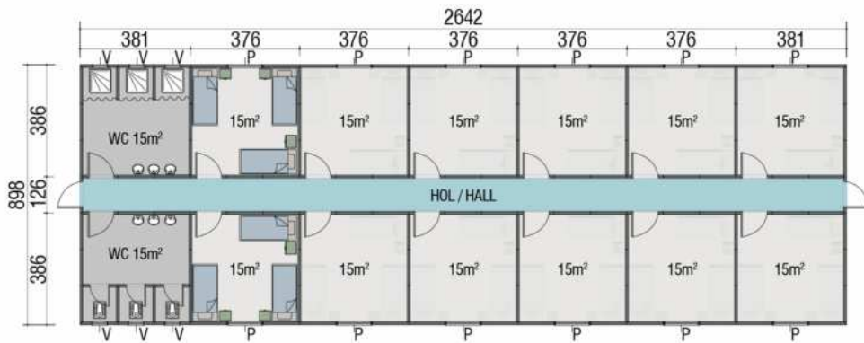
Zemin Kat Planı (237 m 2 ) Ground Floor
